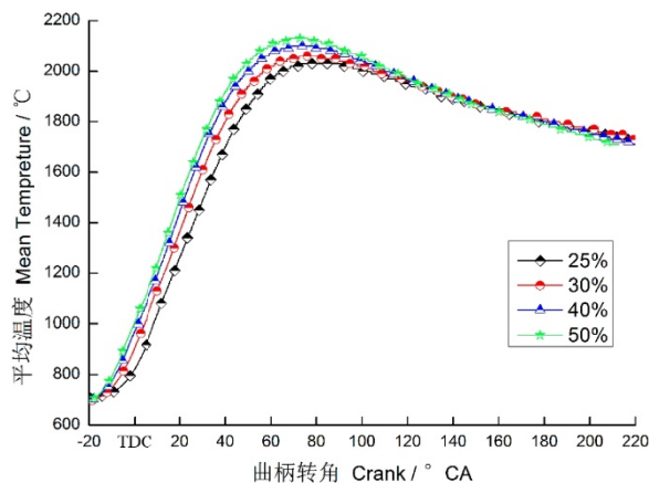
图 7 缸内平均温度
