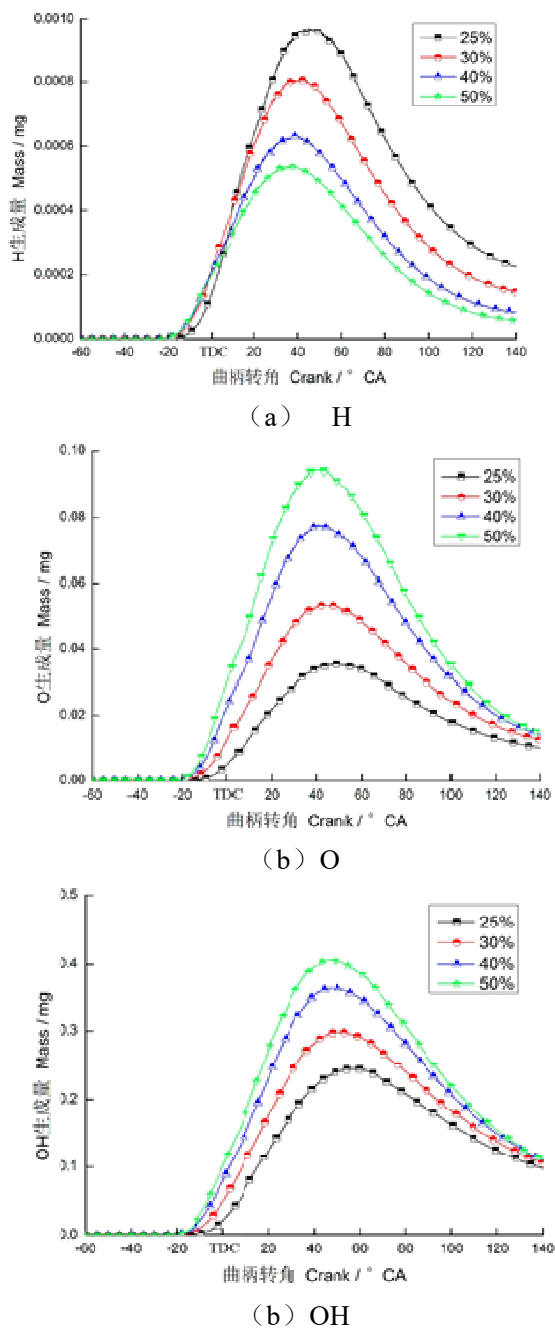
图 8 H、O、and OH 基团的生成量
