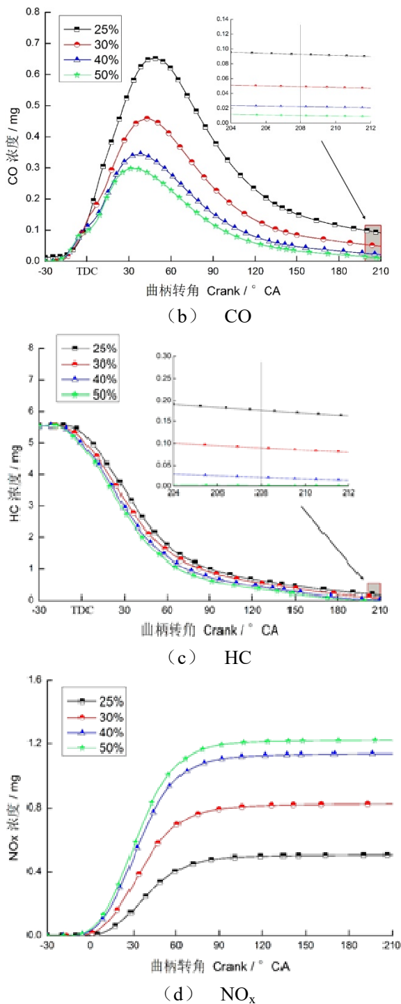
图9 排放物的生成量
