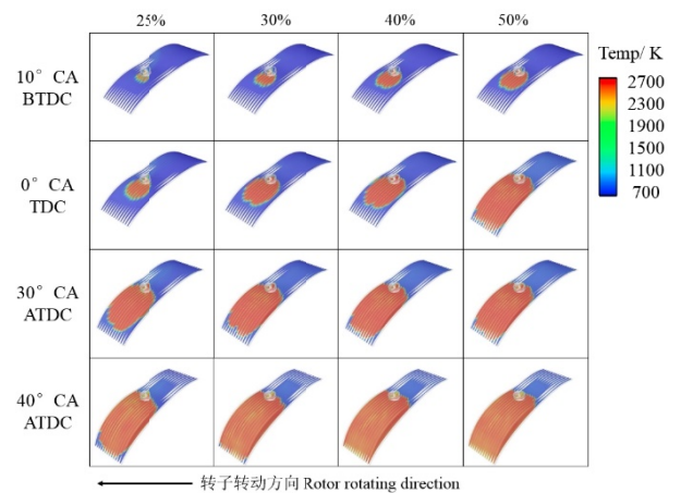
图3 温度场分布
