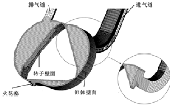
图1 转子机三维网格模型
