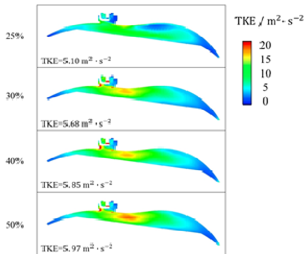
图 5 缸内 TKE 分布(点火时刻)
