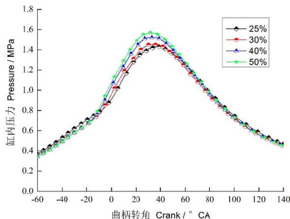
图 6 缸内平均压力
