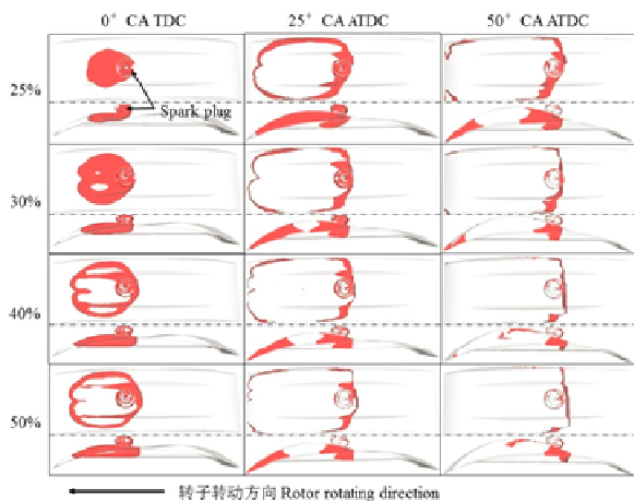
图 4 火焰锋面位置
