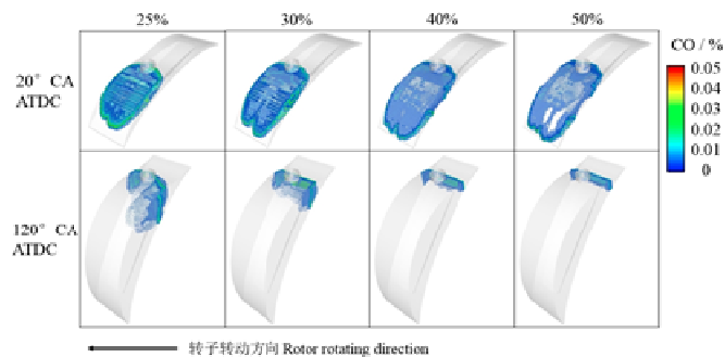
图10 CO 浓度分布
